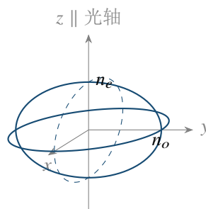
负单轴晶体
