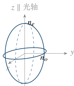
正单轴晶体
