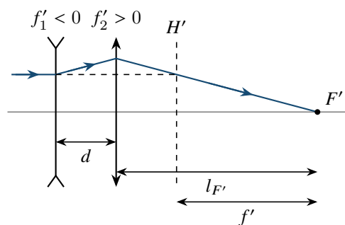
反远距型：后工作距大于焦距
