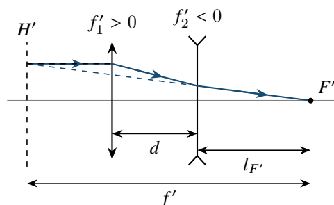
远摄型：像方主面可在前组之前
