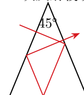
施密特棱镜主截面
