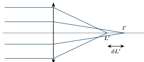
正透镜的负球差
