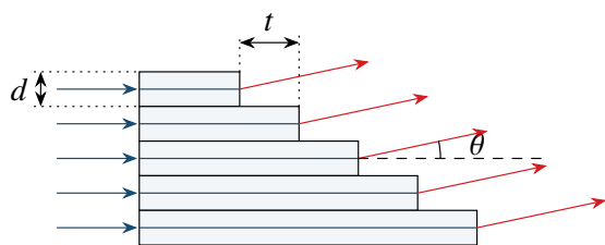
透射型: \theta 向右上为正 入射 \rightarrow 玻璃折射率 n
