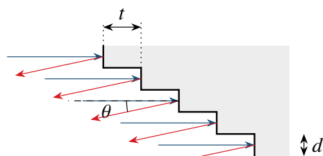
反射型: \theta 向左下为正 入射 \rightarrow 反射 \leftarrow
