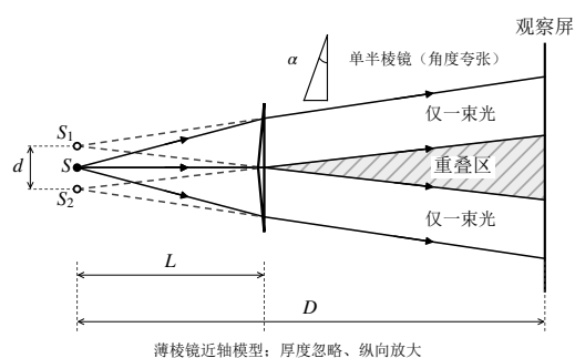
薄棱镜近轴模型: 厚度忽略、纵向放大
