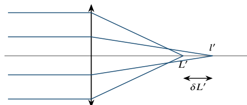
正透镜的负球差
