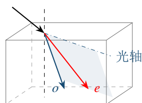
重合: o, e 主平面 与主截面重合
