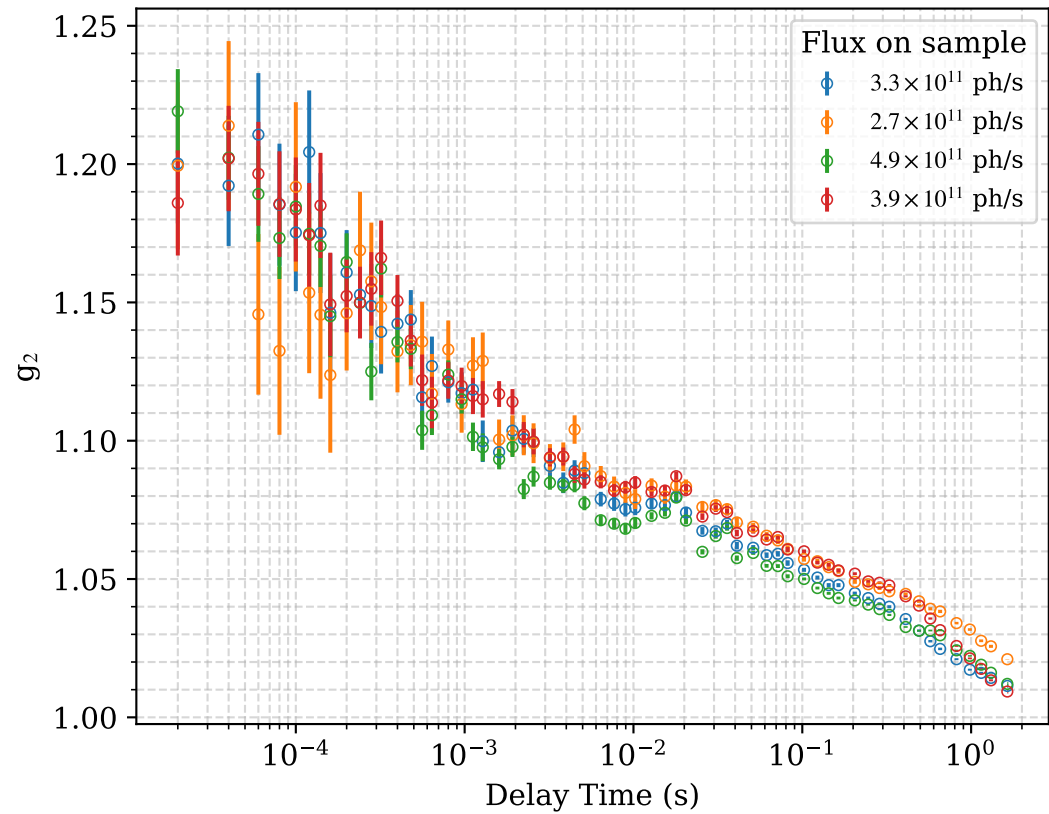
XPCS
