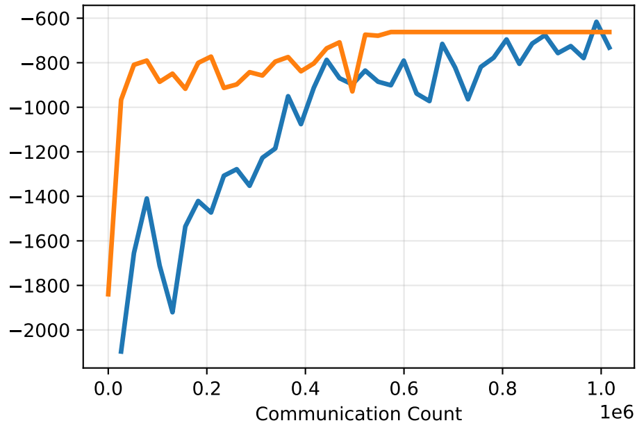
FACMAC
