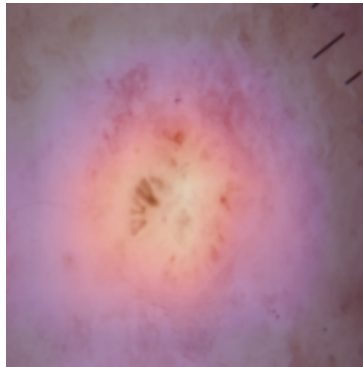
densenet201
