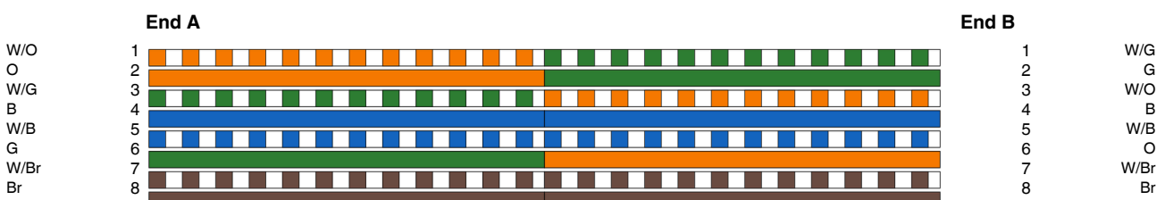
Cable 2: Crossover cable (T568B - T568A)
