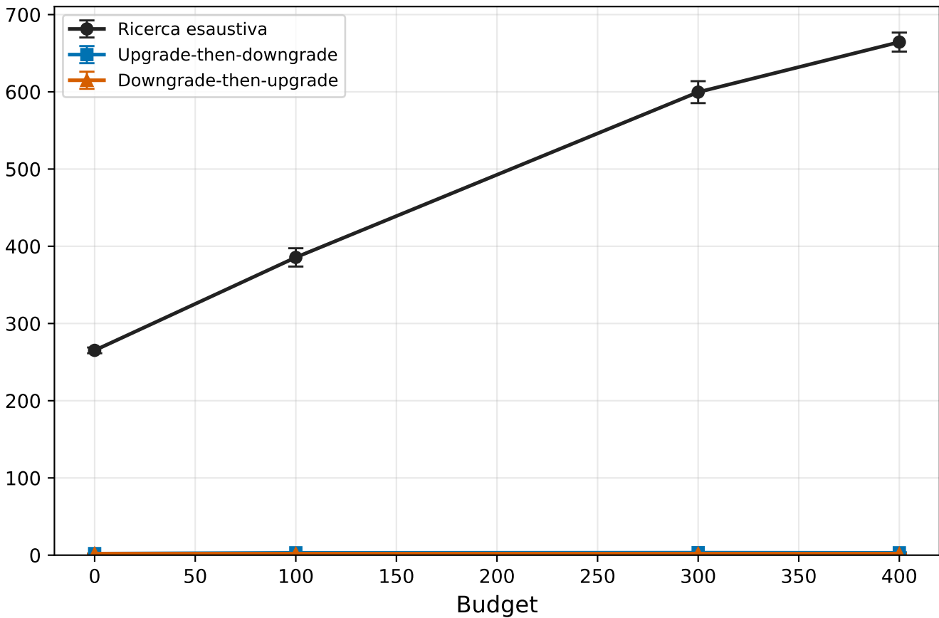
Numero di valutazioni ProbLog
