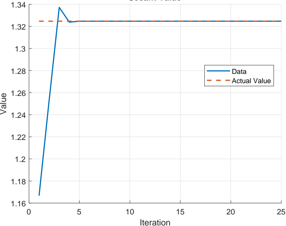
Secant Value
