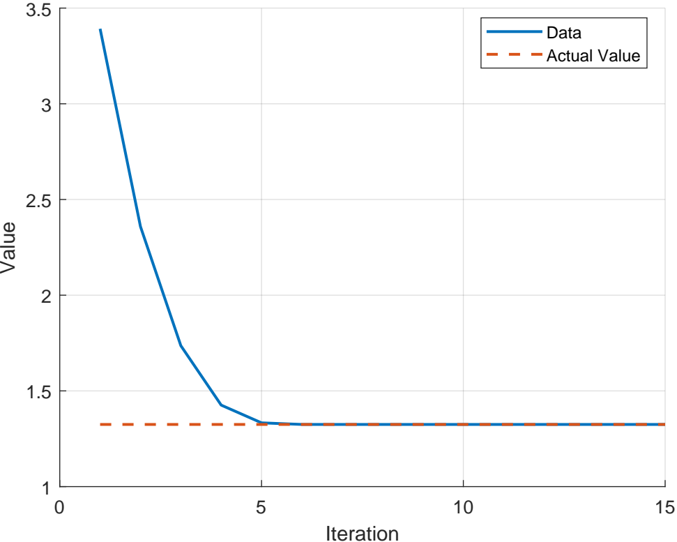
NR Error 1.000000e-14 tolerance
