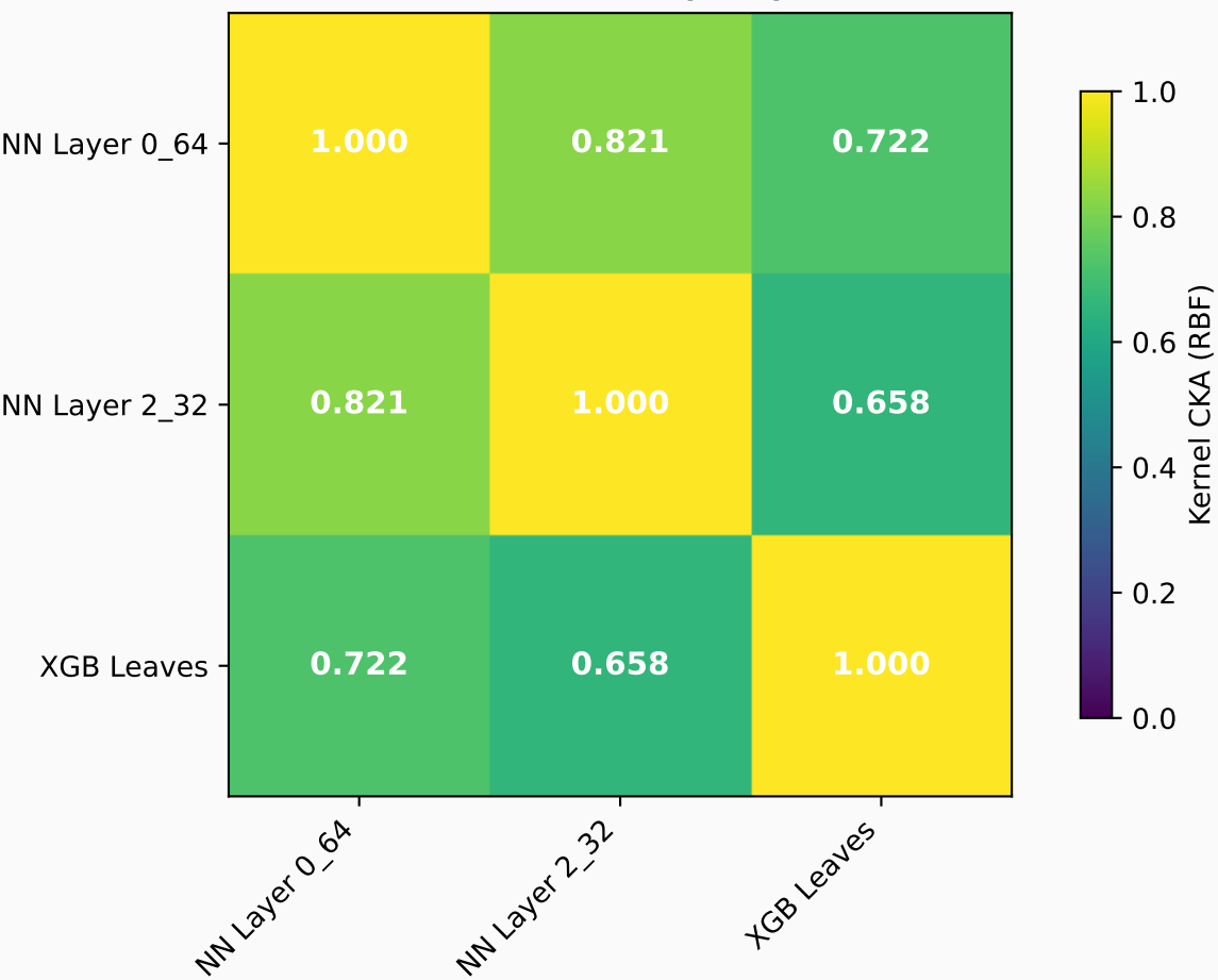
Kernel CKA (RBF)
