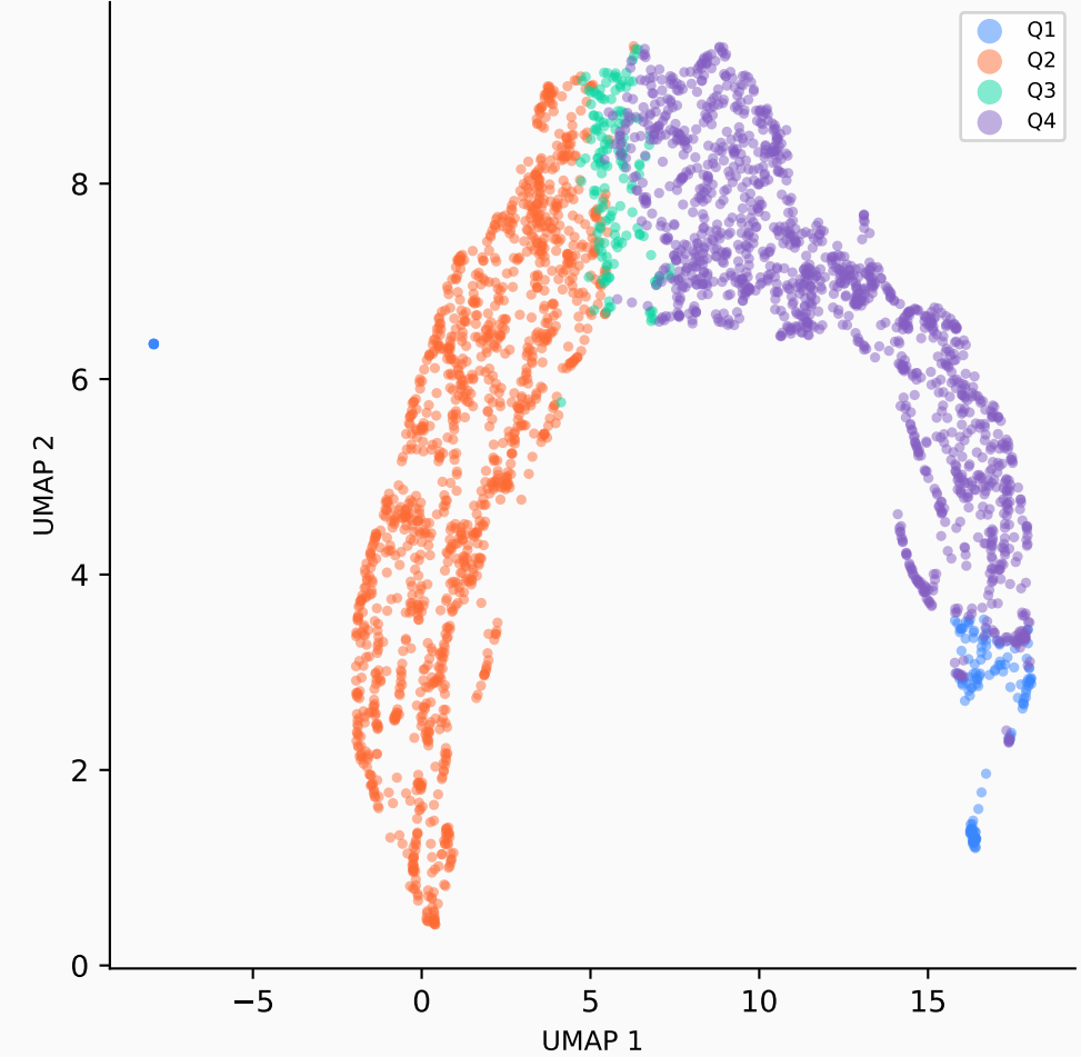
UMAP
