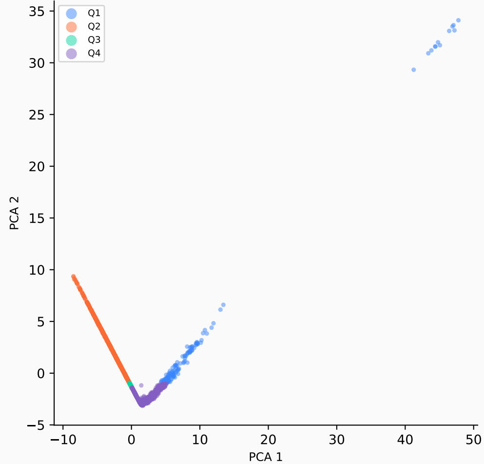
PCA
