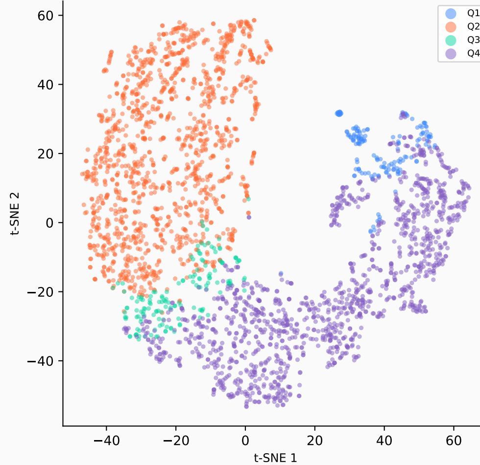
t-SNE
