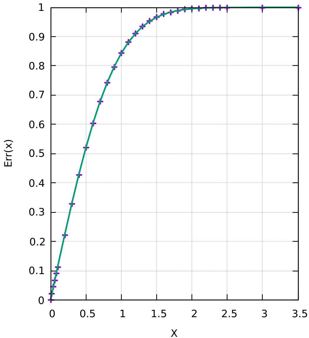
Error function
