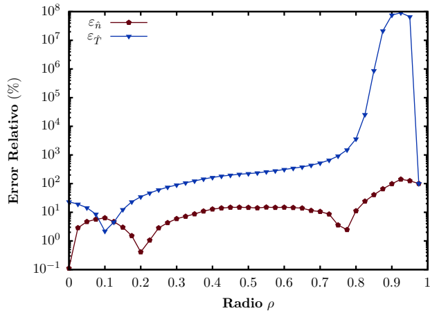
Figura 6: Error relativo entre los perfiles de densidad y temperatura electrónica obtenidos por la PINN en comparación al promedio de las mediciones sobre el RTP.
