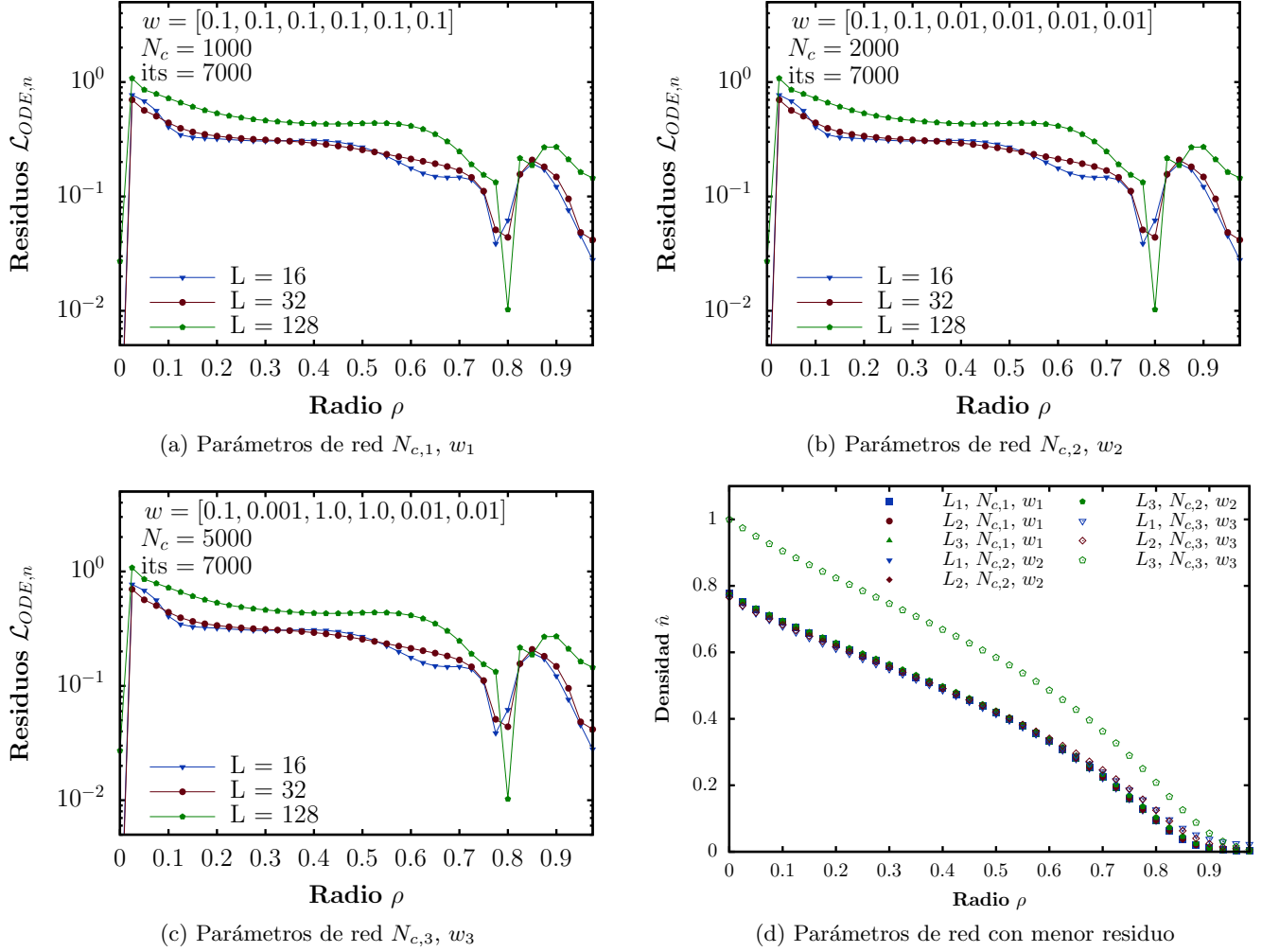
Figura 2: Residuos de la función de pérdida para el ODE de partículas para diferentes números de capas ocultas L para la PINN con: (a) con puntos de colocación N_{c,1} y pesos w_1 , (b) con puntos de colocación N_{c,2} y pesos w_2 , (c) con puntos de colocación N_{c,3} y pesos w_3 y (d) perfiles de densidad electrónica con distintos parámetros de la PINN.
