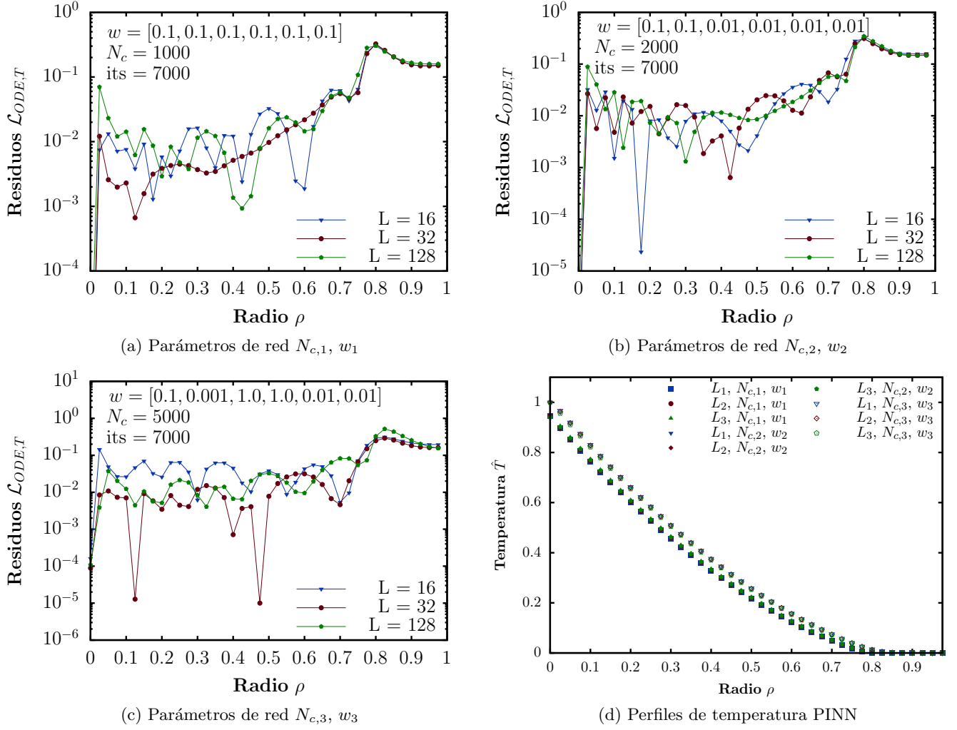
Figura 3: Residuos de la función de pérdida para el ODE de energía para diferentes números de capas ocultas L para la PINN con: (a) con puntos de colocación N_{c,1} y pesos w_1 , (b) con puntos de colocación N_{c,2} y pesos w_2 , (c) con puntos de colocación N_{c,3} y pesos w_3 y (d) perfiles de temperatura electrónica con distintos parámetros de la PINN.
