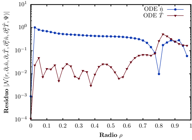
Figura 5: Residuos de la función de pérdida para el ODE de partículas y energía para los parámetros usados que mejor se ajustan a las mediciones.
