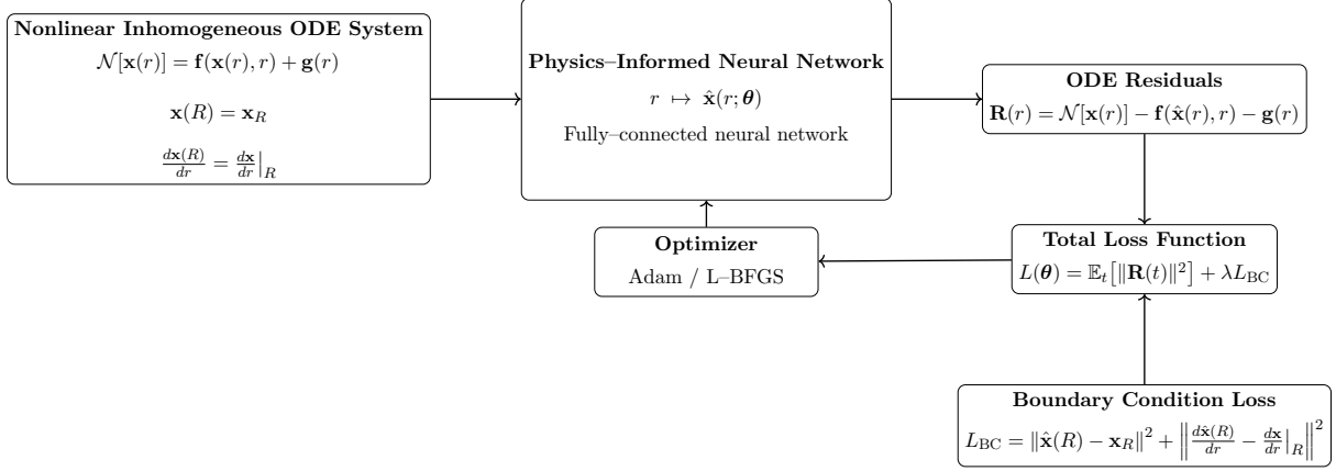
Figure 7: Esquematzación de la implementación de PINNs para la resolución de las ecuaciones (??) y (??) planteadas para el modelo 1D de transporte clásico en un plasma cilíndrico.
