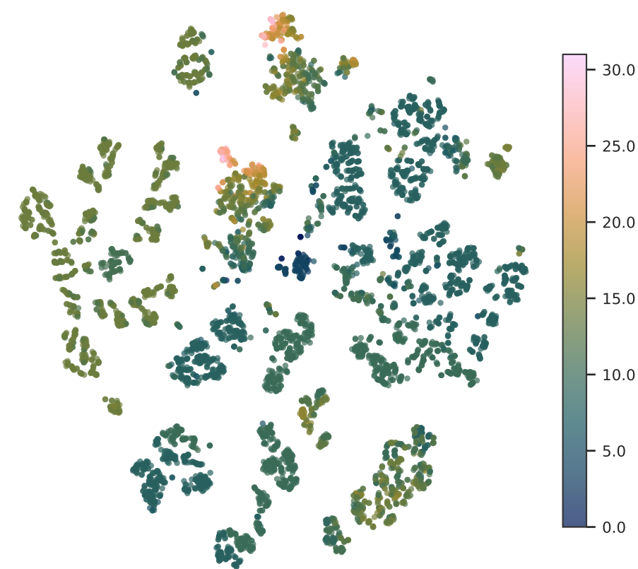
NumRotatableBonds
