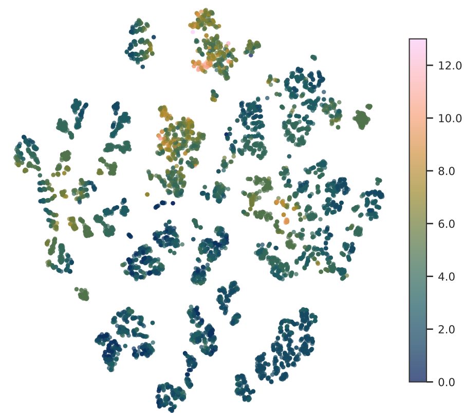
NumHDonors
