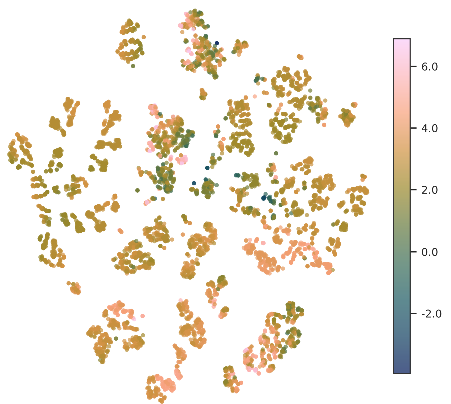
LogP
