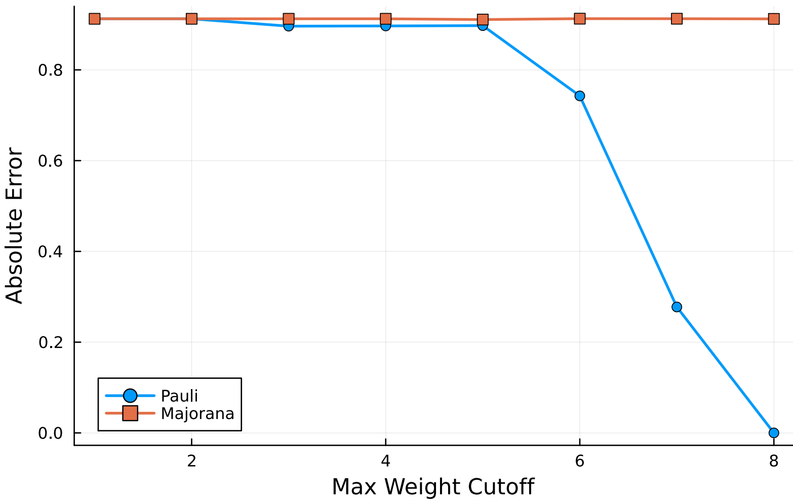
Error vs Max Weight ( N=8 , k=10 )
