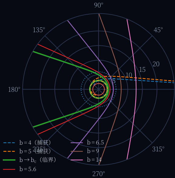
轨道平面内的光子轨迹 r(\phi)
