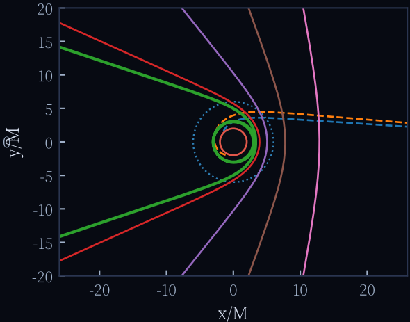
笛卡尔视图 (原点为黑洞)
