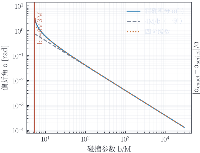
光线偏折角
