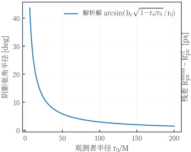
视界阴影的角半径
