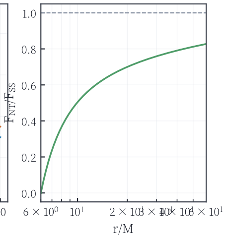
相对论修正 ( r \rightarrow \infty 时 \rightarrow 1 )
