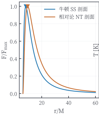
归一化通量剖面
