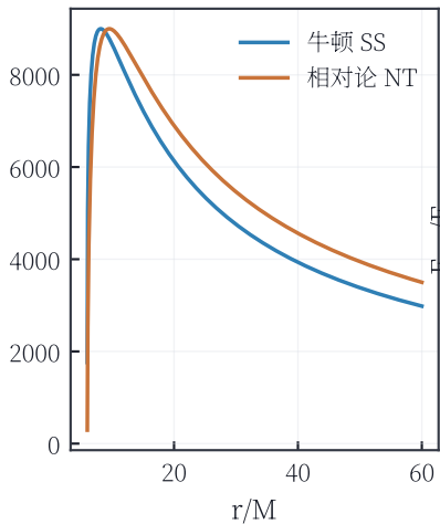
有效温度 T \propto F^{1/4}
