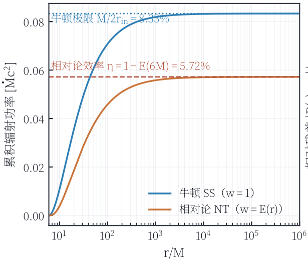
(a) 累积辐射功率 (求和规则)
