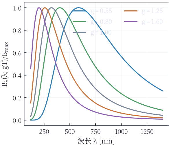
多普勒/引力移动后的黑体谱
