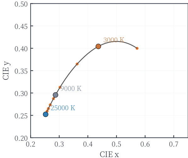
普朗克轨迹与盘色温范围
