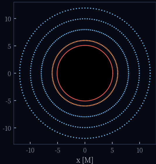
引力透镜化
