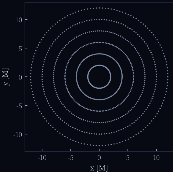
未透镜化
