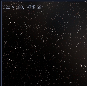
(a) 关闭引力：同一相机的平直时空星场
