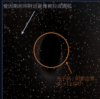
(b) 开启引力： r_0 = 26M 处的透镜化星场
