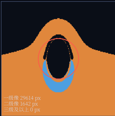
(a) 倾角 i = 8^\circ
