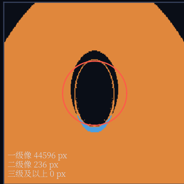
(b) 倾角 i = 55^\circ
