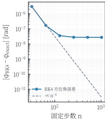
(c) 积分器的四阶收敛
