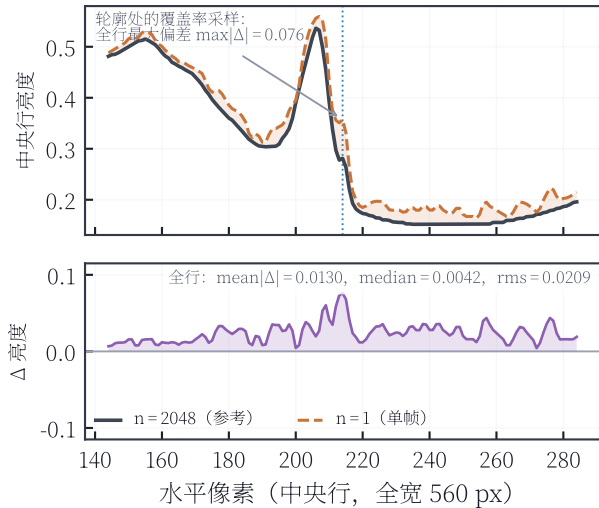
(b) 中央扫描行：单帧 vs 2048 帧
