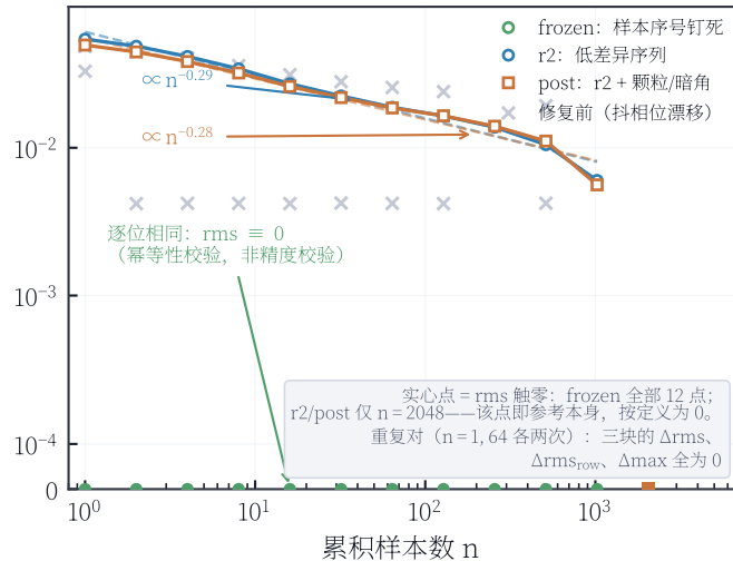
(a) 累积收敛：三条曲线，两种机制
