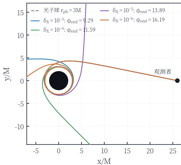
(d) 轨道平面内的环绕: 像阶次的来源 (均自观测者出发)
