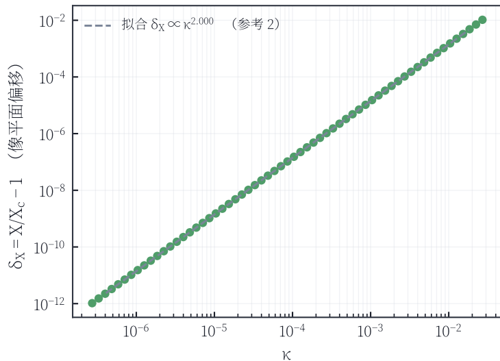
(b) 像平面偏移是 \kappa 的二次映射
