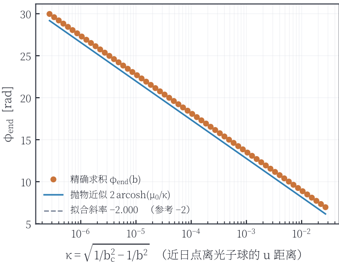
(a) 方位角随 \kappa 对数发散
