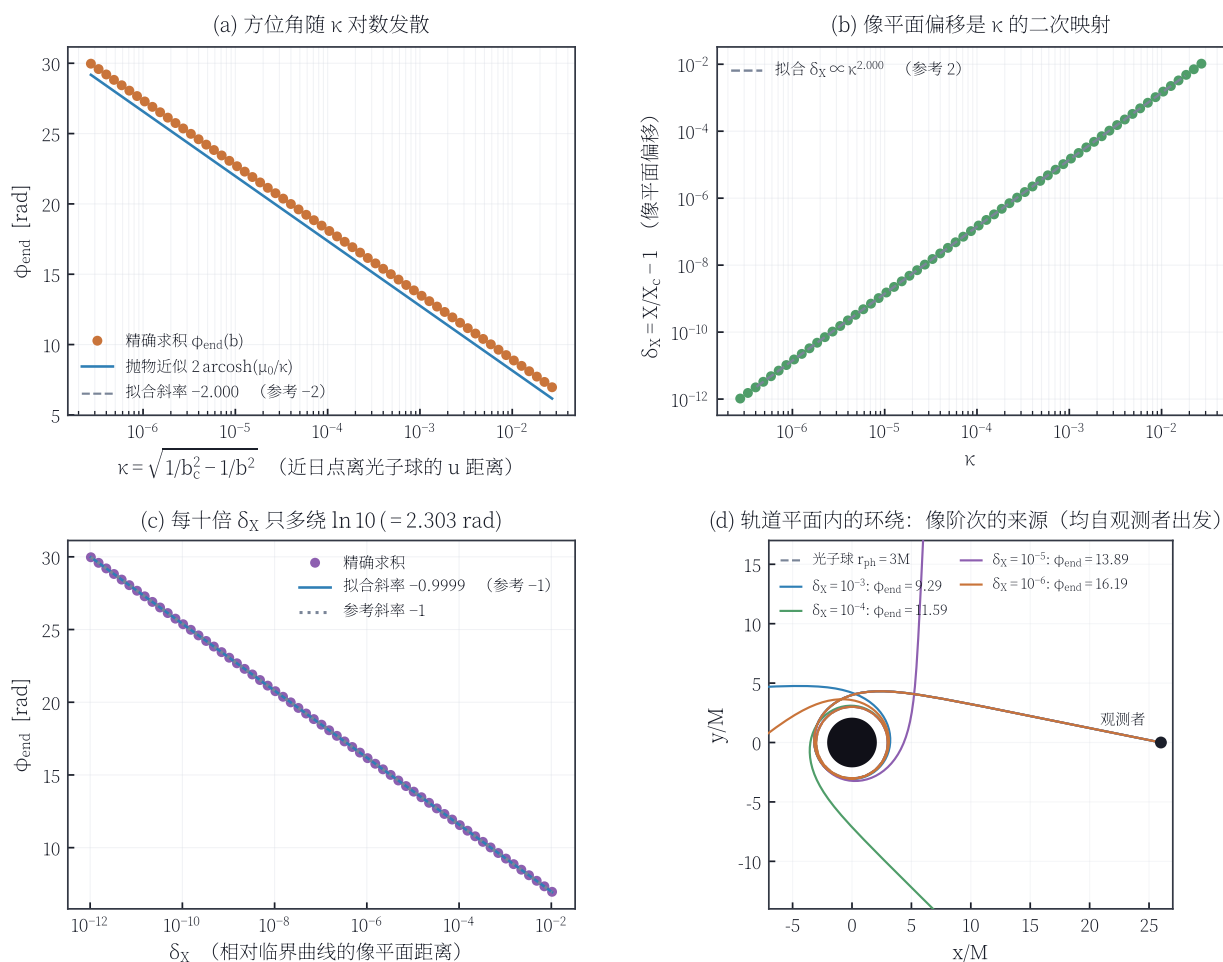
图 14: 近临界光线的对数发散。(a) \varphi_{\text{end}} 对 \kappa = \sqrt{1/b_c^2 - 1/b^2} 的行为 (横轴对数、纵轴线性), 拟合斜率 -1.999946 (参考 -2 ), 虚线为抛物近似 2\text{arcosh}(\mu_0/\kappa) ; (b) 像平面偏移是 \kappa 的二次映射, 拟合指数 2.000059 (参考 2 ); (c) \varphi_{\text{end}} 对 \delta_X 的斜率为 -0.999944 (参考 -1 ), 即每缩小一个量级的像平面距离只多绕 0.37 圈; (d) 轨道平面内的四条近临界轨道 (均自观测者 r_0 = 26M 出发, 虚线为光子球 r_{\text{ph}} = 3M ): 四条曲线出发方向相同, 末端张开的夹角正是 \varphi_{\text{end}} 的对数差异。
