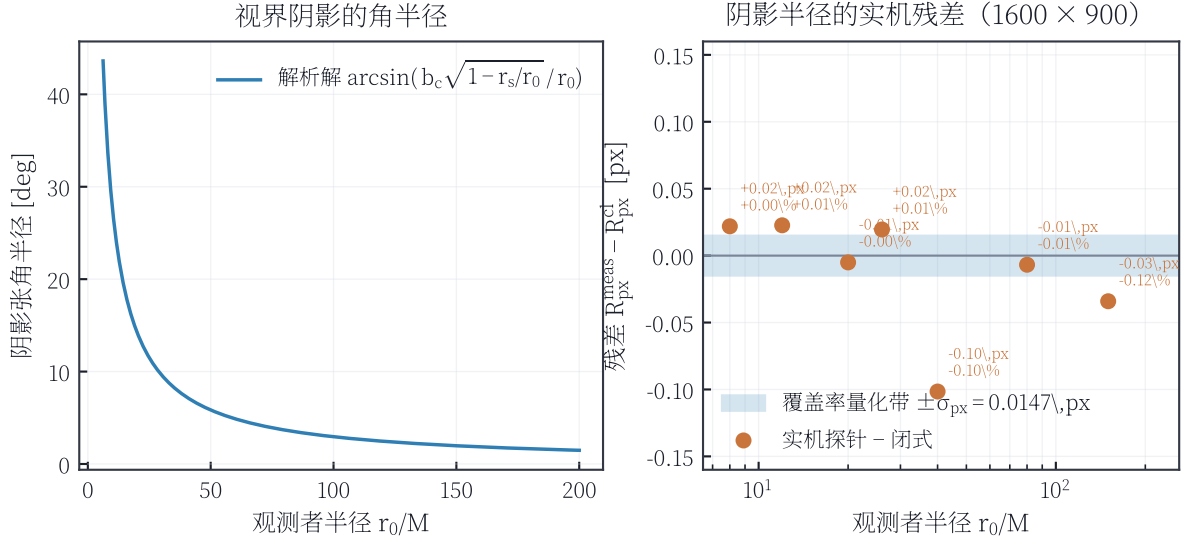
图 17: 阴影半径的两条独立通路。左：闭式 \sin \psi_{sh} = b_c \sqrt{1 - r_s/r_0}/r_0 给出的角半径随观测者半径 r_0/M 的变化 ( b_c = 3\sqrt{3}M )，从 r_0 \rightarrow \infty 处的 \arcsin(3\sqrt{3}M/r_0) 型渐近压到 r_0 = 4M 附近的强场区。右：程序在 1600 \times 900 下实时回读的阴影半径残差（单位为像素），横轴为 r_0/M 。阴影带为 1\sigma 覆盖率量化带 \sigma_{px} = 1/(2\sqrt{2} \cdot 24) = 0.0147 px，每个测点旁标注该点的 \pm 像素残差与 \pm 相对偏差。在修正了式 (64) 中那处把亚像素估计静默退化为整数扫描的钳位之前，同一组测点的绝对残差上界为 0.46 px；修正后降到 0.10 px，即全部测点都落进量化带之内。残差的形状（而不是任何单点数值）是抓到这个缺陷的判据：量化带上界会把残差压成锯齿状，而真实残差应当是平滑的。
