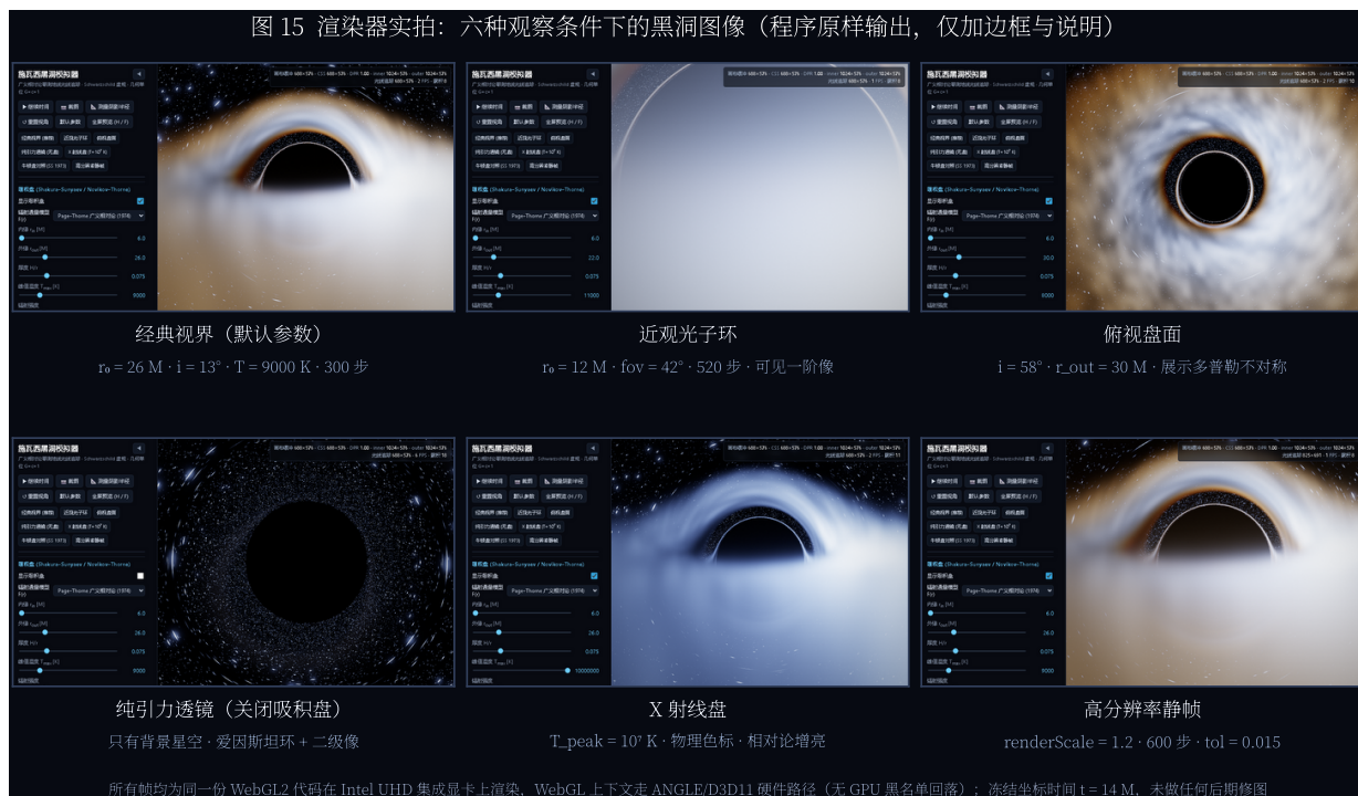
图 15：渲染器实拍：六种观察条件下的黑洞图像（程序原样输出，仅加边框与说明）。所有帧均为同一份 WebGL2 着色器在 Intel UHD 集成显卡上渲染，WebGL 上下文走 ANGLE/D3D11 硬件路径（ANGLE (Intel, Intel(R) UHD Graphics, Direct3D11 vs_5_0 ps_5_0, D3D11)），冻结在 t = 14 \text{ M} ，未做任何后期修图。
