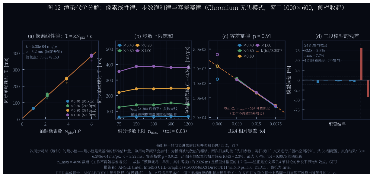
图 12: 渲染代价的三段分解。(a) 像素线性律 T = kN_{\text{pix}} + c : 四个缩放 \times 三轮重复，拟合给出 k = 6.298 \times 10^{-4} \text{ ms/px} 、 c = 5.22 \text{ ms} ；(b) 步数上限的饱和：以 n_{\text{max}} = 300 为基准的归一化耗时在 [0.895, 1.089] 内，300 步之后不再有系统趋势；(c) 容差幂律 T \propto \text{tol}^{-p} ，实测 p = 0.91 ；(d) 三段模型的残差与四个被 n_{\text{max}} = 4096 截断的 \text{tol} = 0.0075 点（空心）。图注中「论文第 7.4 节」即本文 §7.4，那里用同一批数据讨论计时量化。
