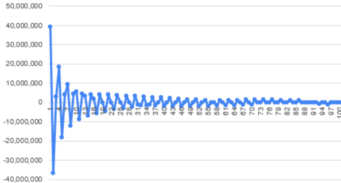
Figura 3.9. Gráfica generada en Excel a partir de los datos exportados por el programa en C, que muestra la magnitud de los términos hasta 100 iteraciones.
