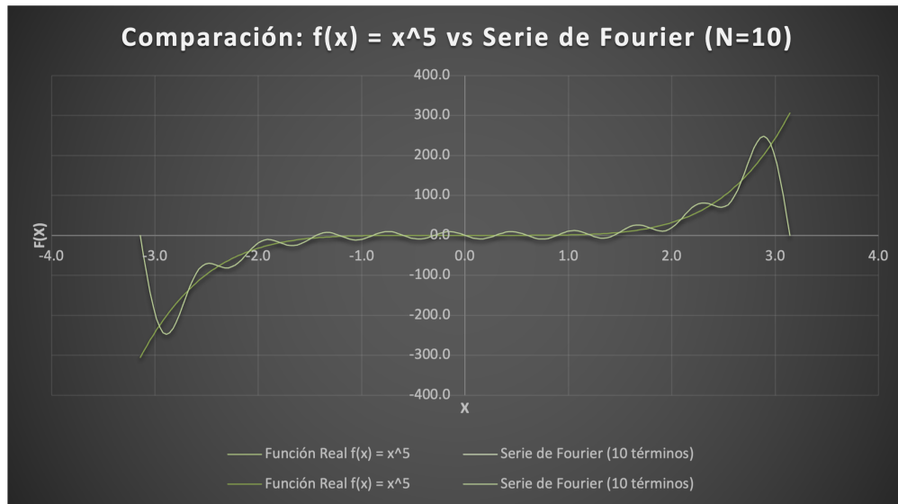
Figura 3.17. Resultados de la fase 2 (capítulo 2): gráfica de la serie de Fourier calculada en Excel con un número reducido de términos ( N = 10 ).
