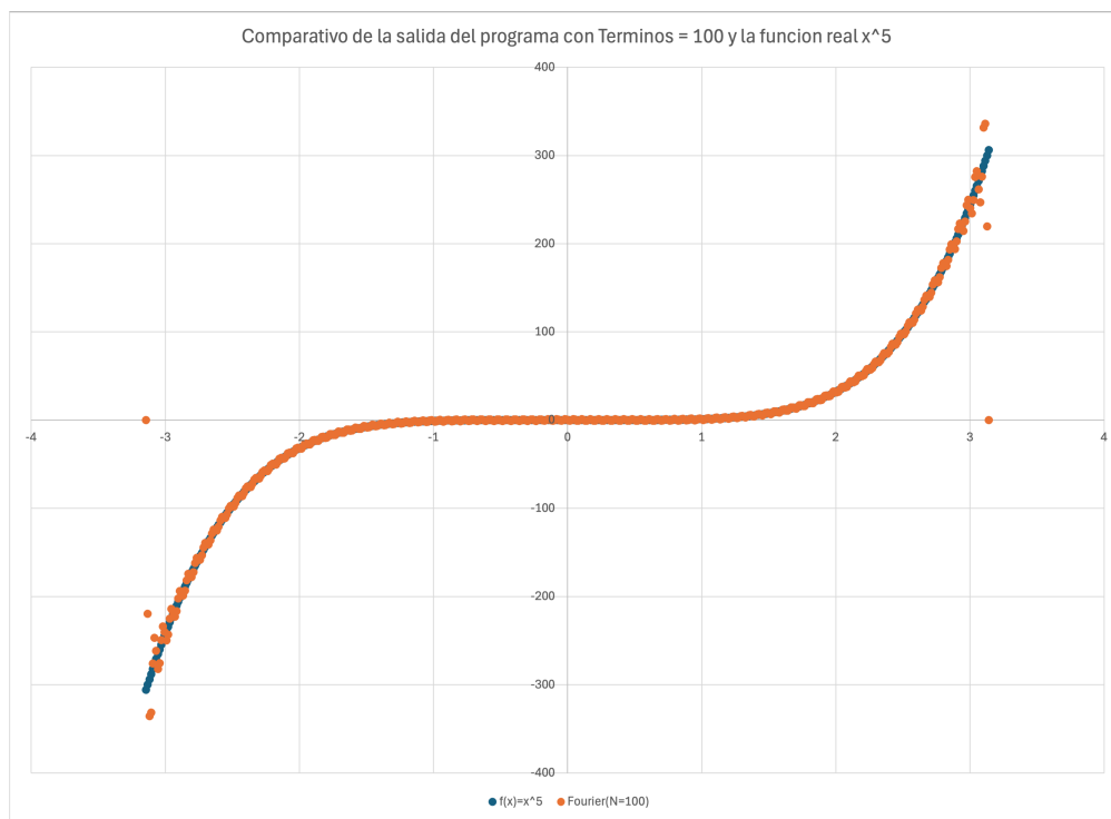
Figura 3.18. Resultados de la fase 3 (capítulo 3): gráfica de la serie de Fourier procesada en lenguaje C con 100 procesos concurrentes.
