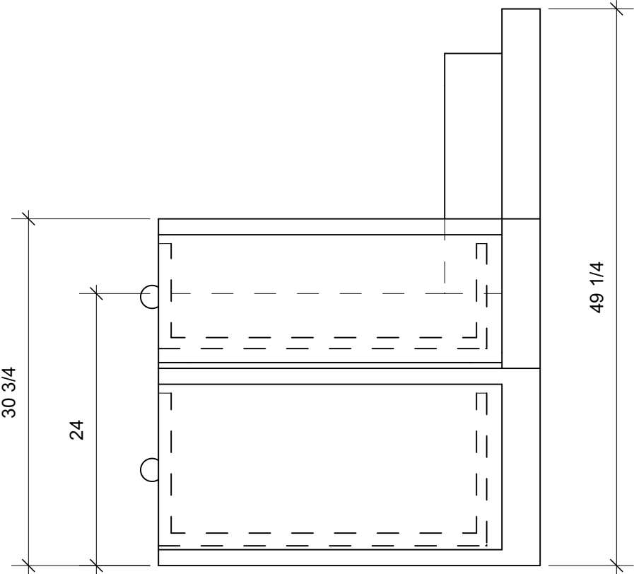
3 RIGHT VIEW Scale: 1" = 1'-0"
