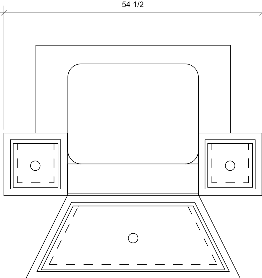
2 FRONT VIEW Scale: 1" = 1'-0"
