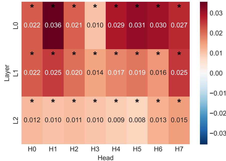
PenDigits (* = FDR p < 0.05 )
