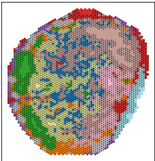
FULL_IGE seed 0
