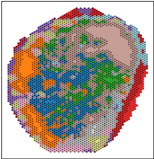
FULL_IGE seed 2
