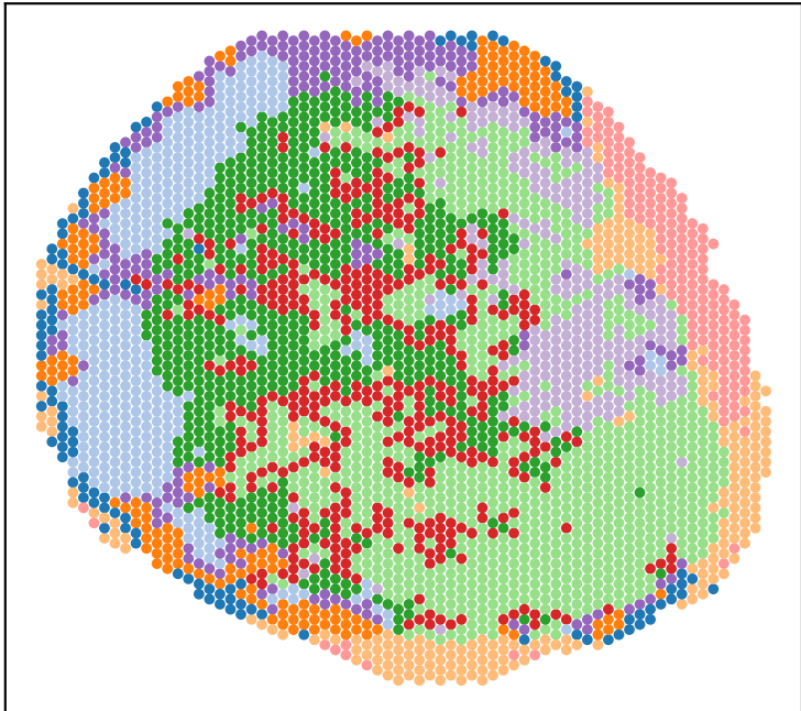
FULL_IGE seed 0
