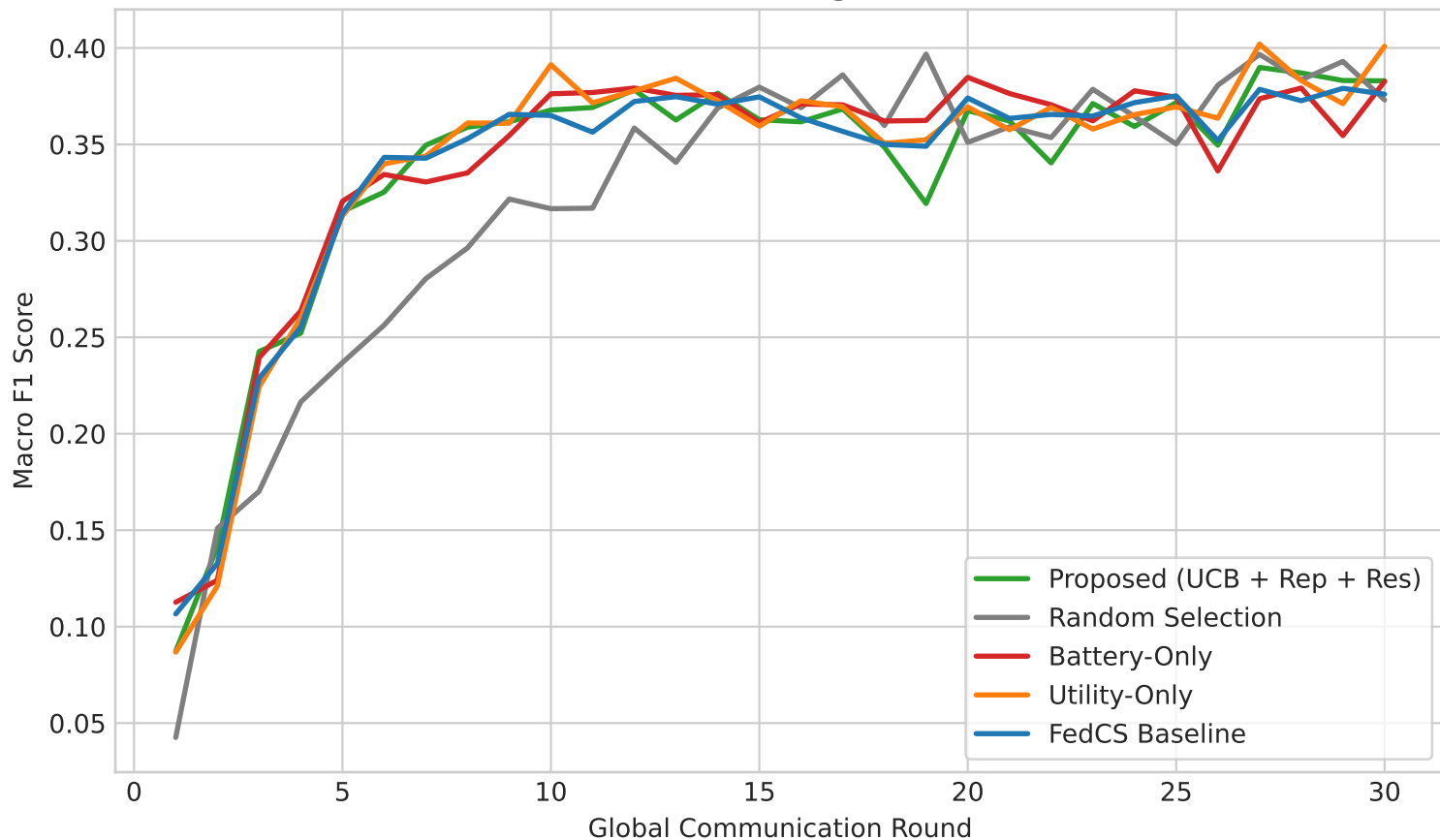
Global Model Macro F1 Convergence (IoT Clients N=14)
