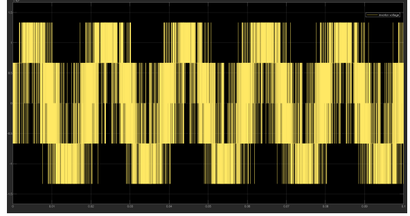
(d) Inverter Phase Voltage
