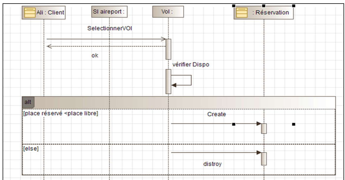
Figure 2 : digramme de séquence du CU «réserver un vol ».
