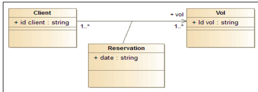
Figure 1: digramme de classe « système de réservation de vol »
