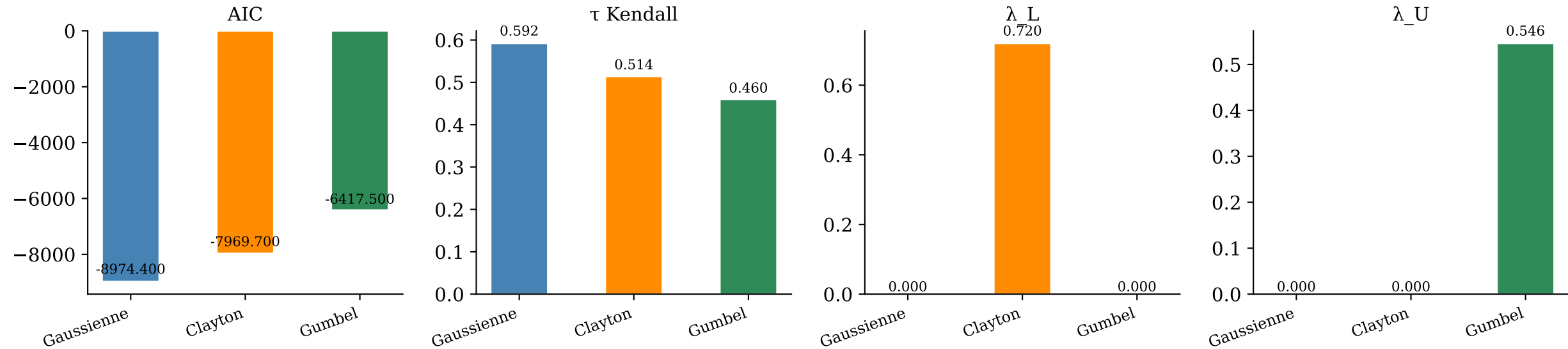
Figure 6.2 — Comparaison des copules | Résidus EGARCH, 2025
