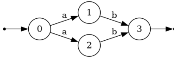
FIGURE 4 – Automate après suppression des transitions epsilon
