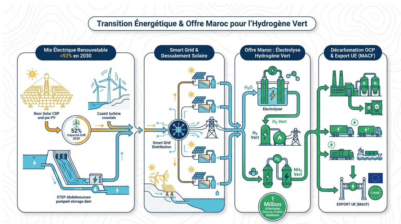
FIGURE 2-2 – Mix électrique renouvelable (objectif 52%) et filière hydrogène vert au Maroc
