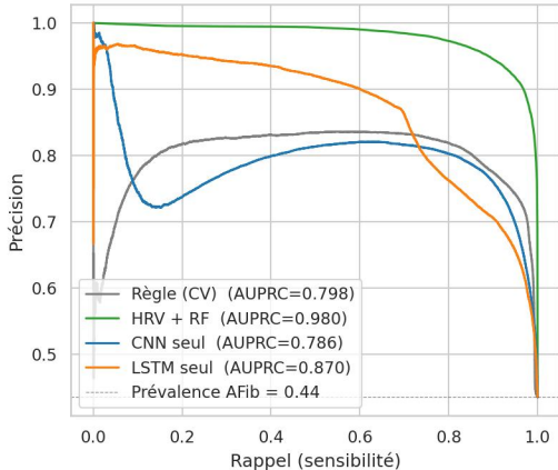
Courbes Précision-Rappel — OOF AFDB 5-fold patient
