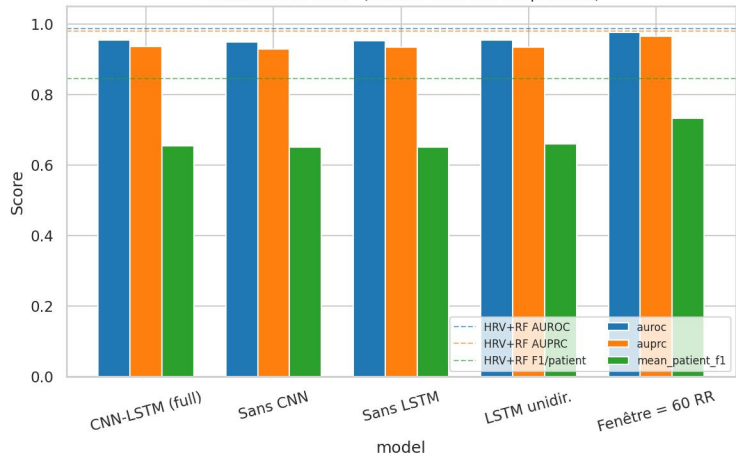
Ablation CNN-LSTM (vs floor HRV+RF en pointillé)
