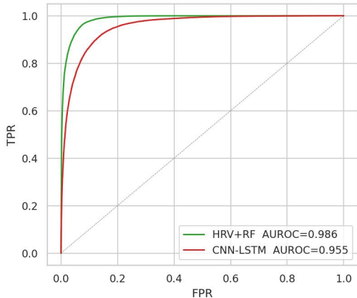
ROC — HRV+RF vs meilleur CNN-LSTM
