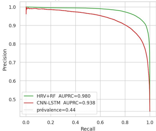
Précision-Rappel — HRV+RF vs meilleur CNN-LSTM
