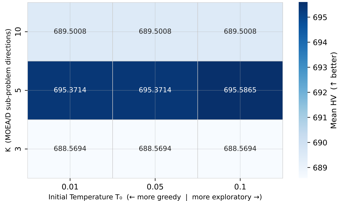
HV Heatmap — w: 0.7 → 0.3 Eyeriss / CIFAR-10 / 300 NFE / 3 seeds
