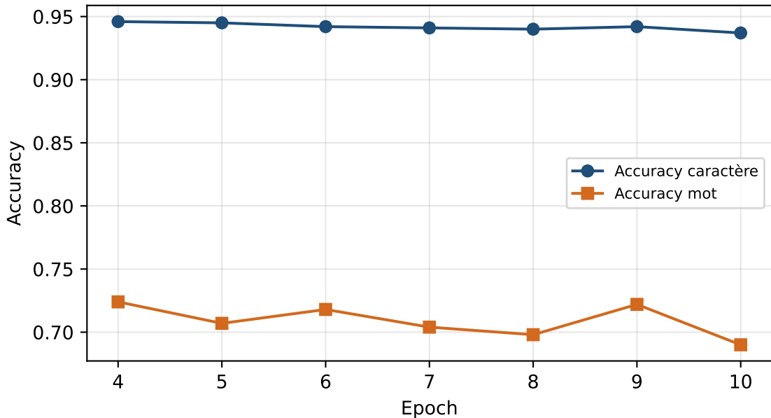
Précision caractère et mot (validation) par epoch
